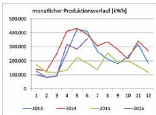
Der monatliche Produktionsverlauf des E-Werks unterliegt starken Schwankungen. In den Monaten der Schneeschmelze sowie im November erreicht die Stromproduktion die höchste Leistung, in den Monaten Dezember bis März erreicht sie ihren Tiefststand (Skizze: Ing. Georg Untergassmair).
